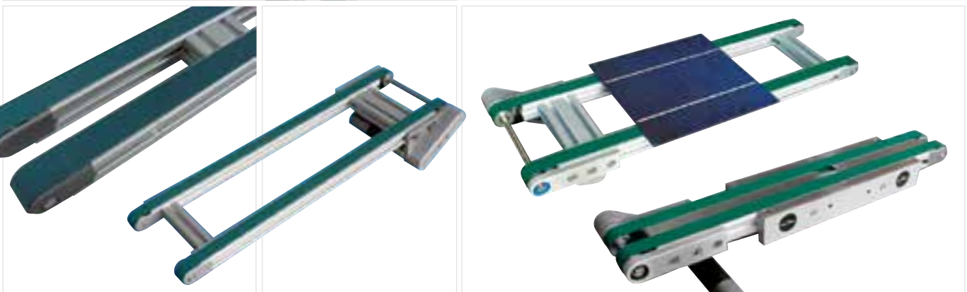
Kit BK-20 con Accionamiento indirecto.
